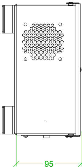
Вид зліва
