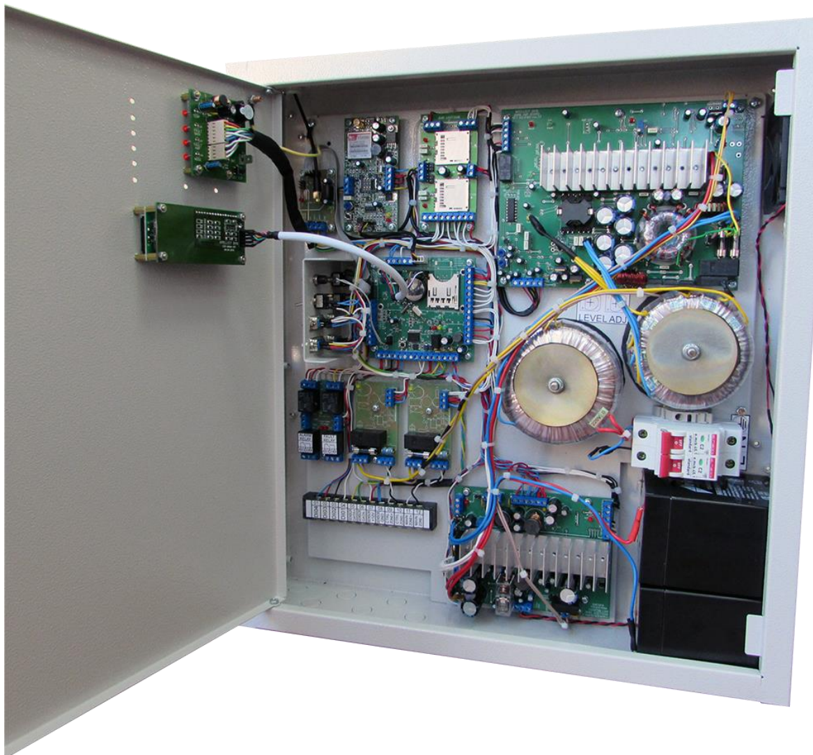
Загальний вигляд моноблоку СОЛА 21 з відкритими дверцятами
