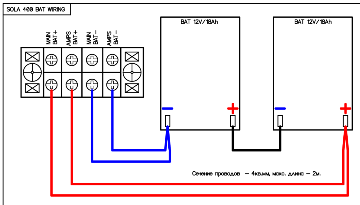
Малюнок 5.3.1 Схема підключення батареї СОЛА 400Вт
